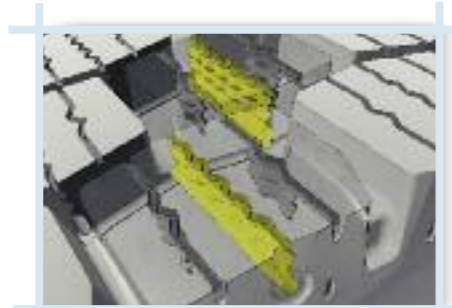
Samouzamykací „dvojitá lamela“ zvyšuje tuhost dezénových bloků, zajišťuje vyšší záběrovost a vysoký kilometrový výkon.
