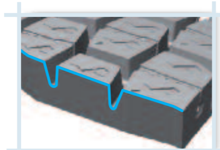
Nový tvar dezénu zamezující zachytávání kamenů.
